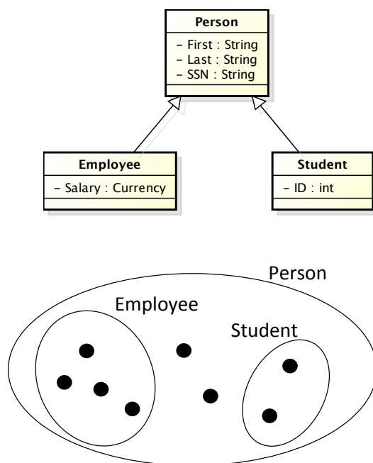
Figura 4.12: Rappresentazione della generalizzazione o specializzazione
