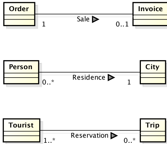
Figura 4.8: Esempi di molteplicità
