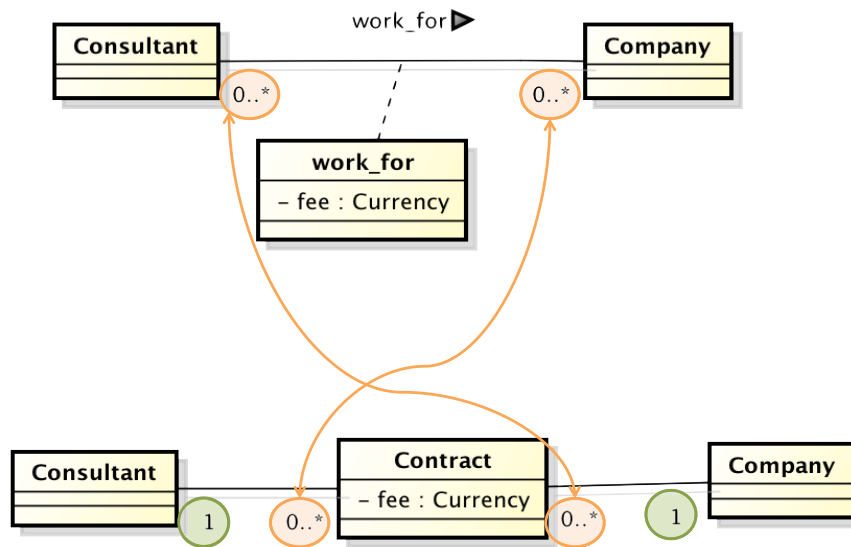
Figura 4.10: Classe di associazione e classe intermedia
