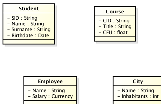
Figura 4.3: Rappresentazione grafica degli attributi
