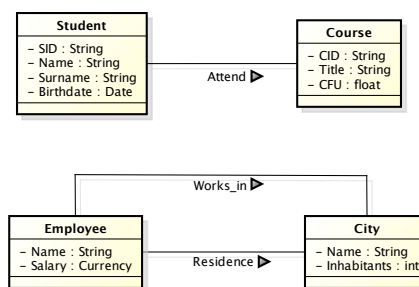
Figura 4.5: Rappresentazione grafica delle associazioni
