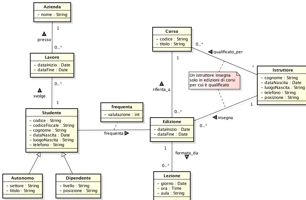
Figura 4.17: Terzo raffinamento del modello
