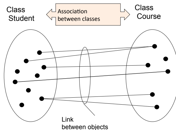
Figura 4.4: Associazioni e link
