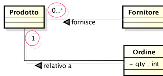
Figura 4.14: Obbligatorietà delle associazioni
