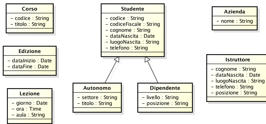
Figura 4.16: Secondo raffinamento del modello
