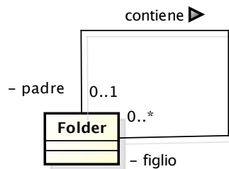
Figura 4.15: Gearchia tramite associazione ricorsiva
